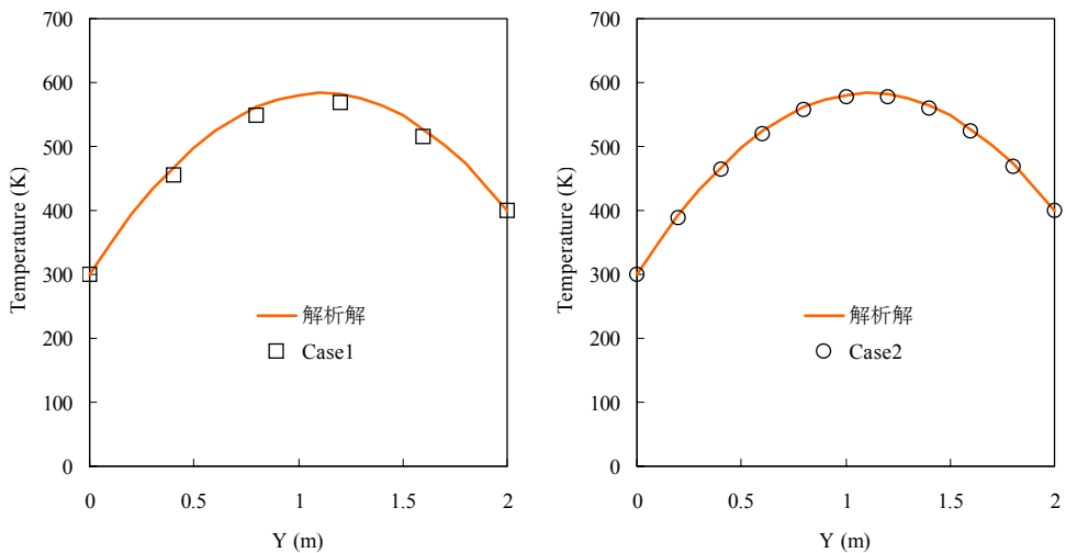
図 1-2 解析解と計算値の温度分布の比較
