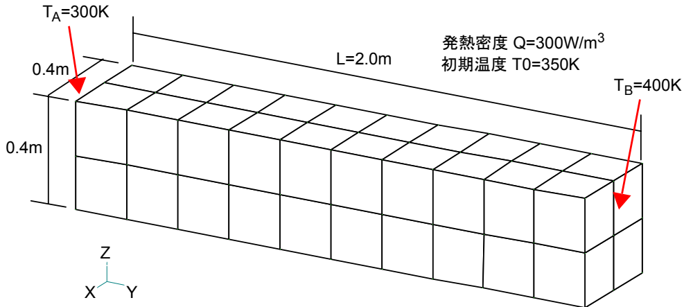
図 1-1 計算モデル
